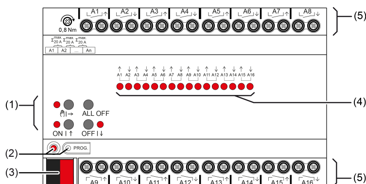
Afbeelding 1: Constructie apparaat
