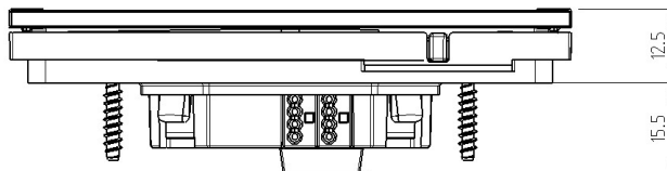
Bild 7: Einbaumaße
