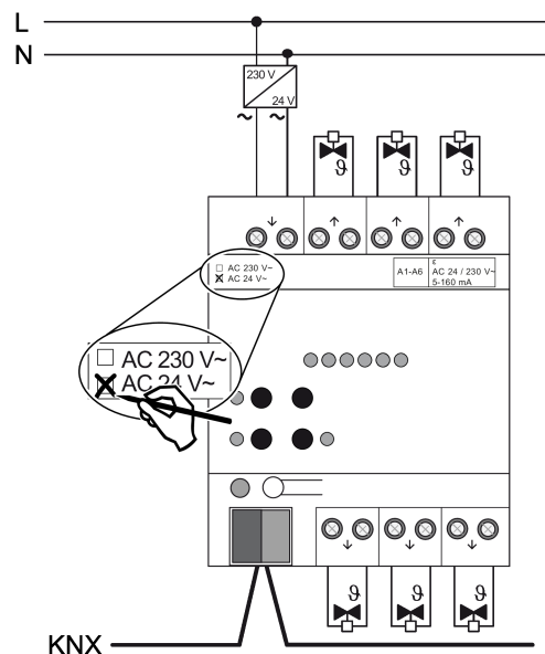
Imagen 4: Conexión de accionamientos reguladores 24 V
