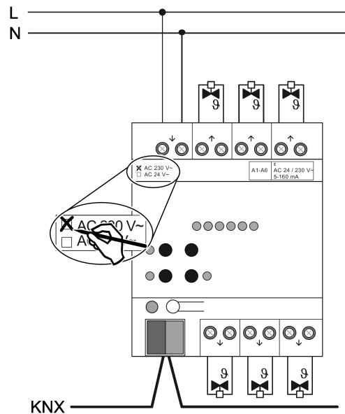
Imagen 3: Conexión de accionamientos reguladores 230 V
