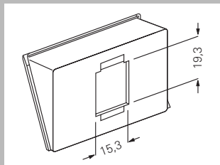
Inzetstuk voor Modular Jack/Western Techniek AMP/Radiall, 1voudig 0052 00
