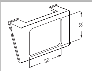
Inzetstuk voor AMP/ACO (Communications Outlet) Alleen geschikt voor 30° uitgang. 0059 00
