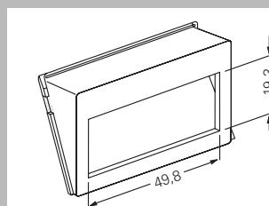
Inzetstuk voor Modular Jack/Western Techniek AMP, 2voudig 0039 00
