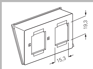
Inzetstuk voor Modular Jack/Western Techniek AMP/Radiall, 2voudig 0053 00
