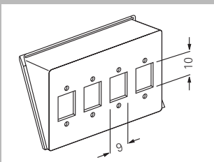
Inzetstuk voor glasvezelkabel/ SC-Duplex-koppeling, 4voudig 0090 00
