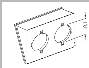
Universeel inzetstuk 0049 00
