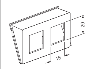
Inzetstuk voor System Thomas & Betts (Nevada Western Structured Wiring System/IBM ACS Mini-C/600 MHz) 0064 00
