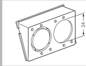
Inzetstuk voor twee XLR-ronde stekerver- bindingen, C-serie 0092 00
