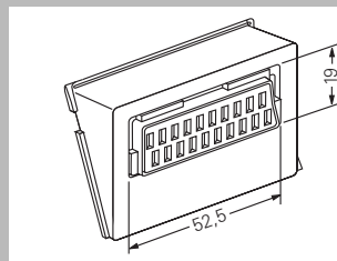
Inzetstuk met Scart/Euro-AV-bus 0093 00
