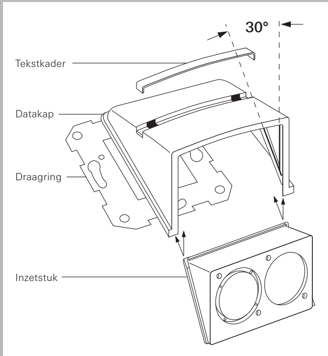
Datakap voor data- en communicatie-aansluitingstechniek
