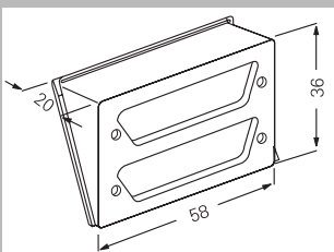
Inzetstuk voor D-subminiatuur 0050 00
