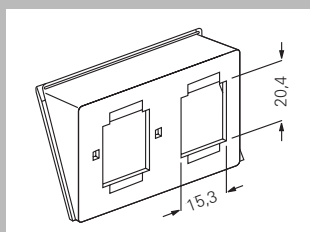
Inzetstuk voor Modular Jack/Western Techniek AMP, 2voudig 0039 00
