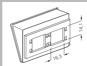
Inzetstuk voor Modular Jack/Western Techniek AMP/Radiall, 2voudig 0053 00
