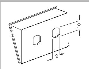
Inzetstuk voor ST-glasvezelkabel 2,5 mm 0732 00
