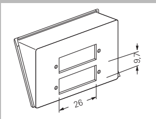
Inzetstuk voor glasvezelkabel/ SC-Duplex-koppeling, 2voudig 0089 00
