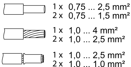
рисунк 2: Зажимаемое поперечное сечение провода
