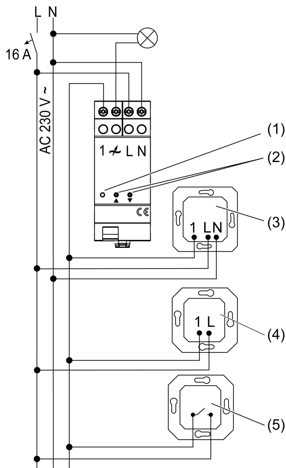
Bilde 1: Koblingskjema
