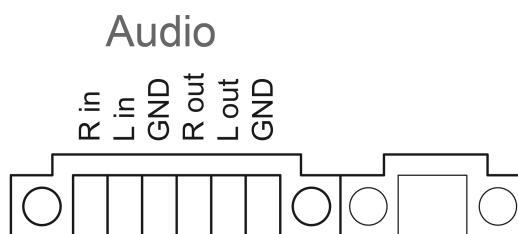
Bilde 6: Tilkoblingskonfigurasjon audioforbindelser
